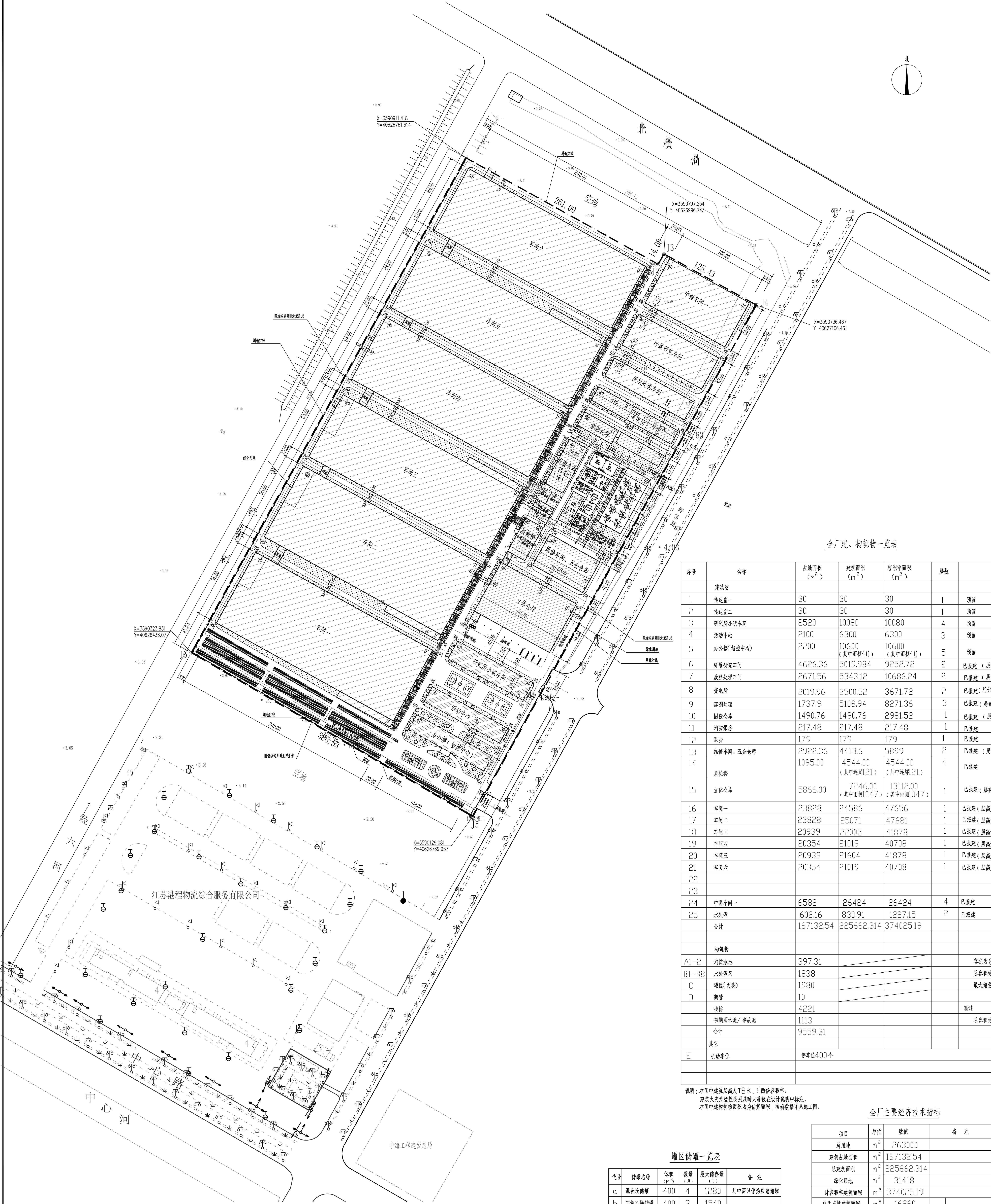
总平面布置图 1:1500
