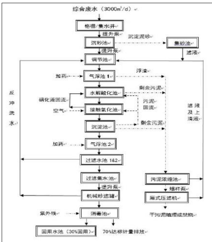
图 3.1.2-1 原大豫镇加工区污水处理厂工艺流程图
