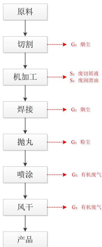
图 5.2-3 智能制造典型工艺流程及产污环节图
