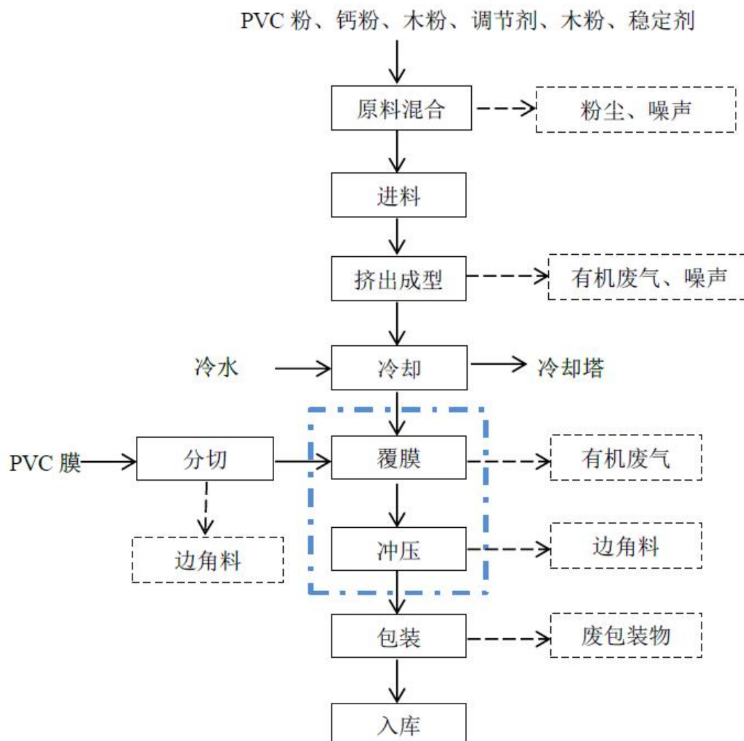
图 5.2-4 装饰装修材料典型工艺流程及产污环节图
