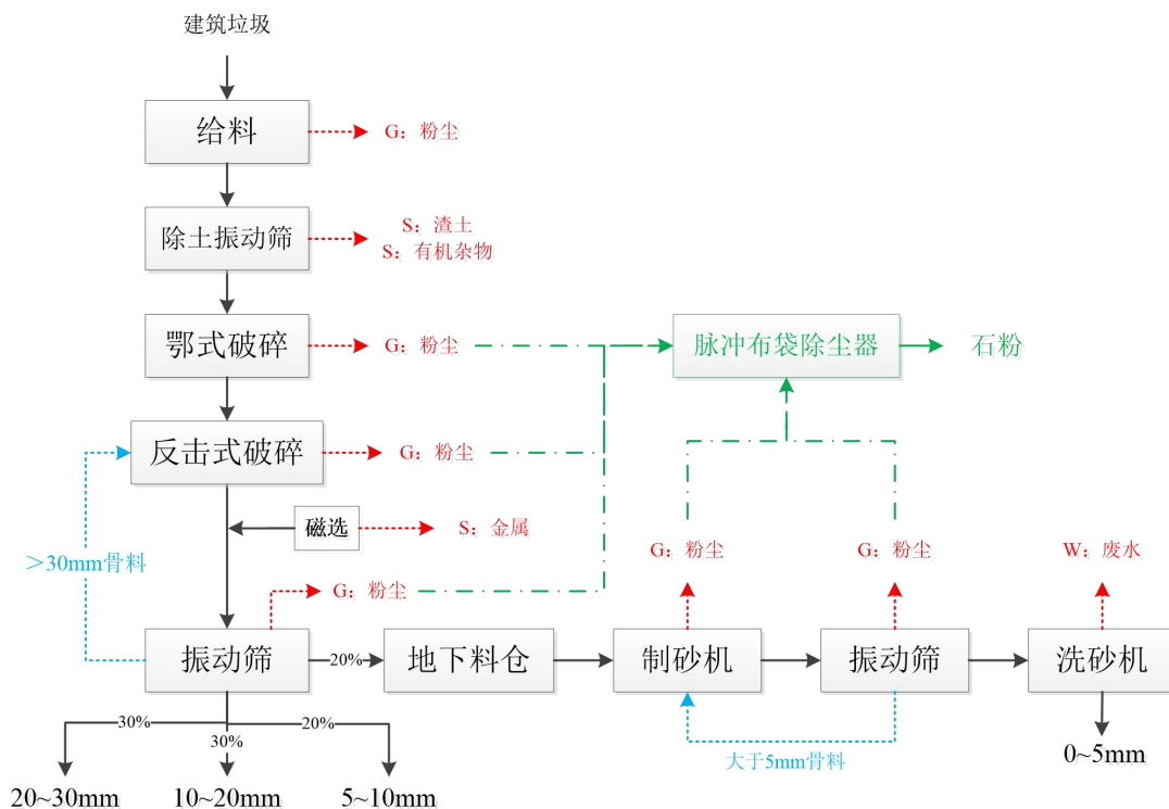
图 5.2-2 拆迁垃圾综合利用典型工艺流程及产污环节图
