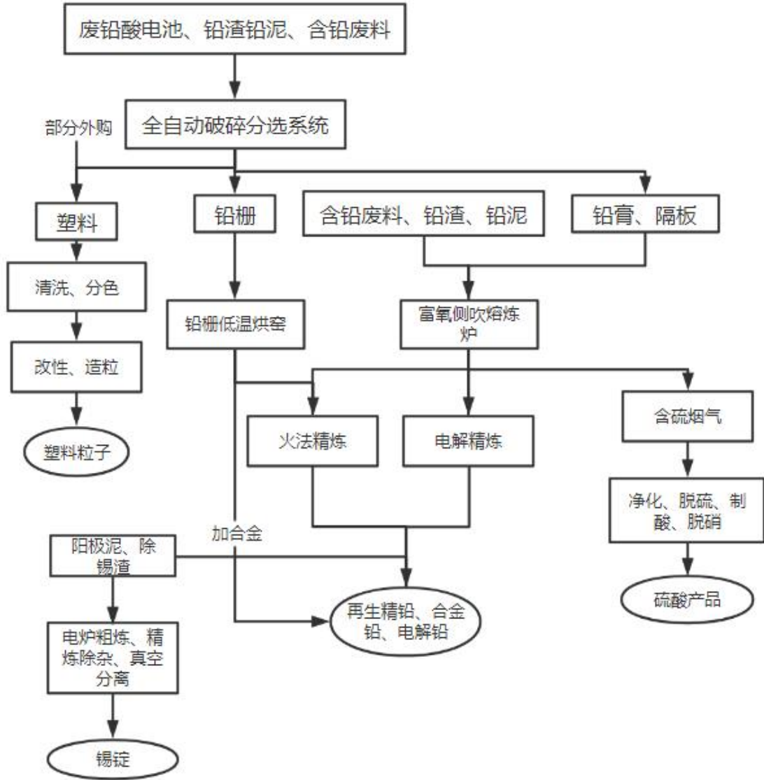
图 5.2-1 废铅酸电池综合利用典型工艺流程及产污环节图
