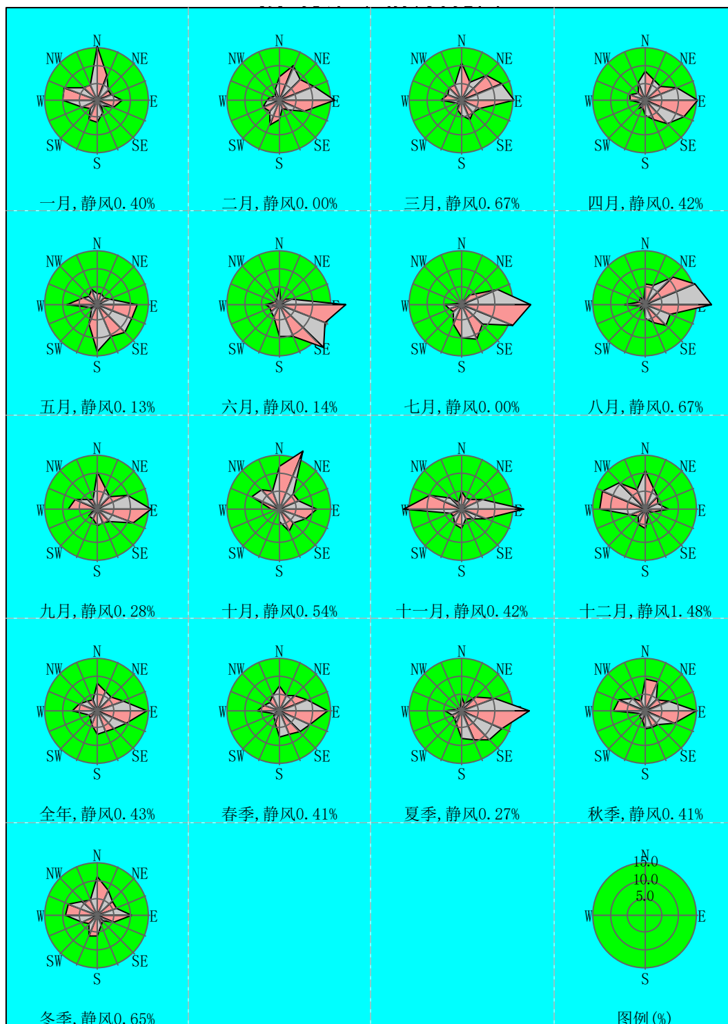
图 6.1.2-2 2021 年各月份、季度及全年风向玫瑰图
