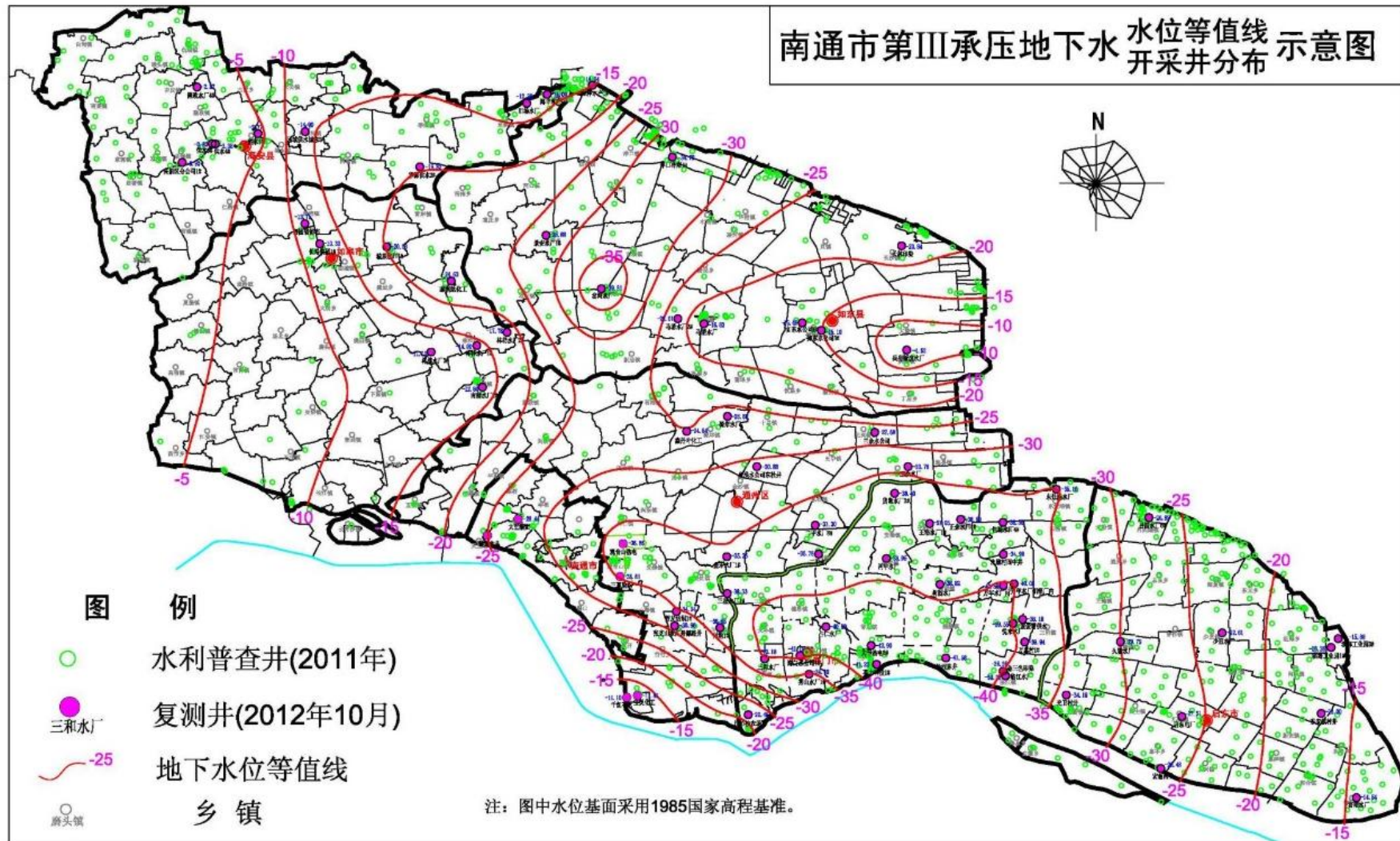
图 6.4.2-2 第Ⅲ承压地下水水位等值线示意图
