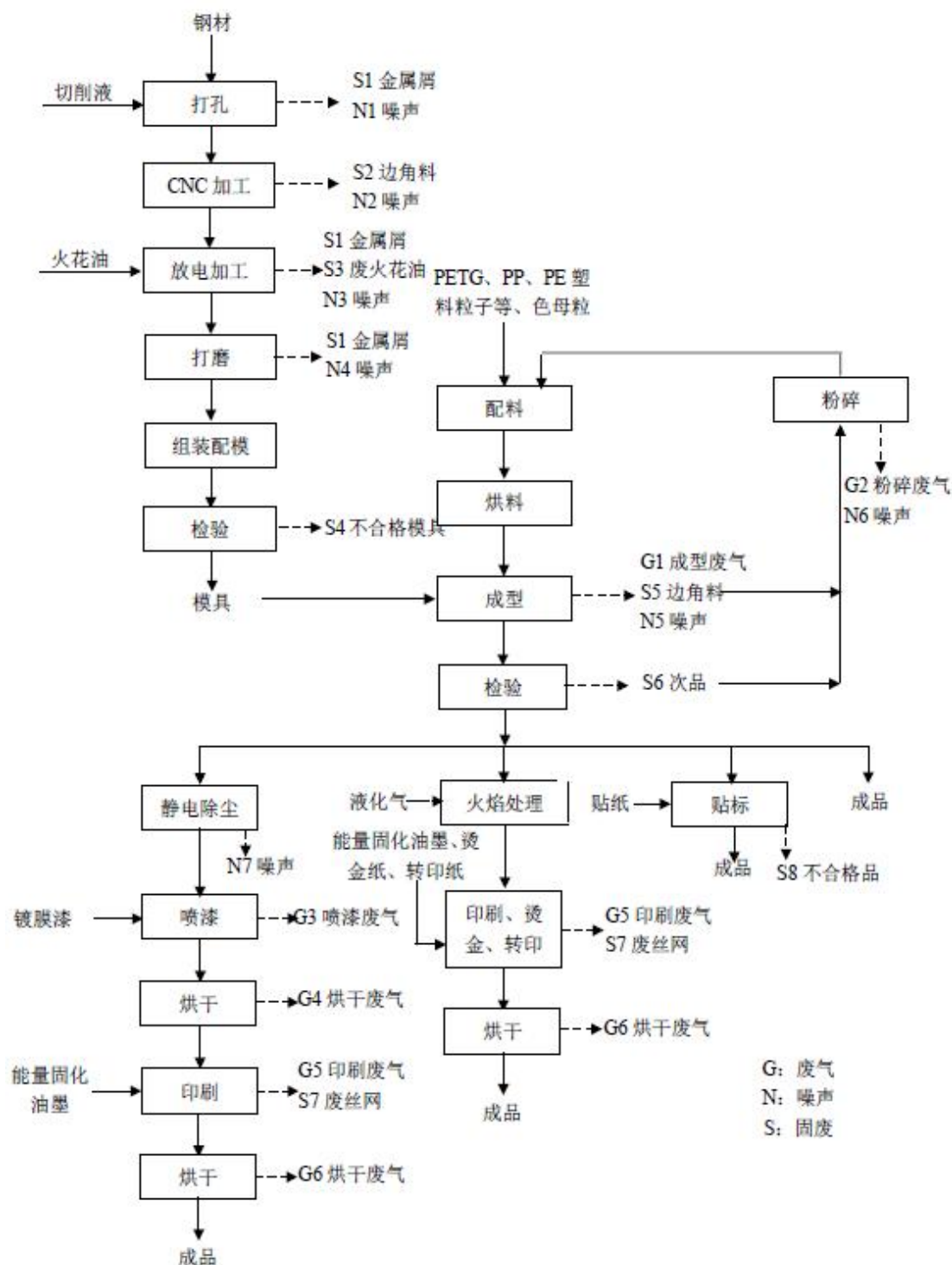
图 5.2-6 橡胶和塑料制品典型工艺流程及产污环节图
