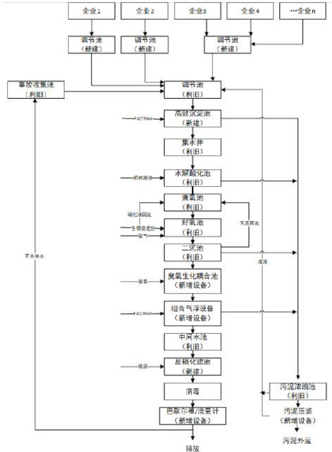
图 6.2.2-1 提标改造后污水处理工艺流程图
