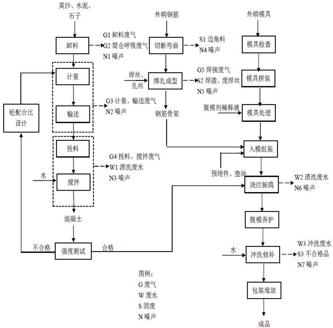
图 5.2-5 装配式构件典型工艺流程及产污环节图
