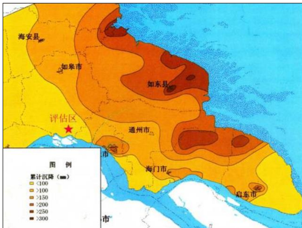
图 6.4.3-2 南通地区地面沉降分布图
