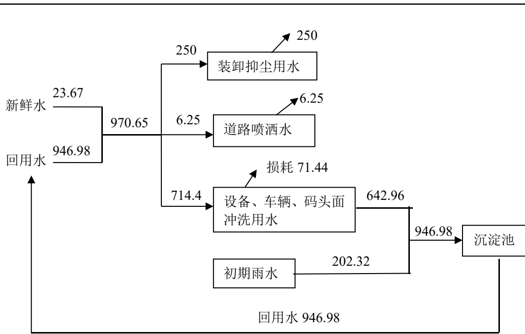
图 4-1 本项目水平衡图 t/a
