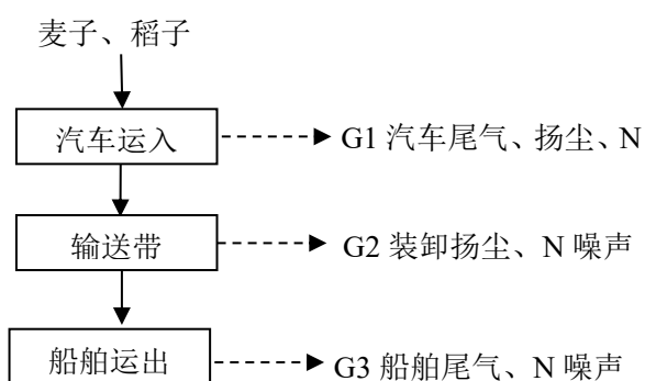
图 2-1 麦子、稻子装卸工艺流程及产污环节图
